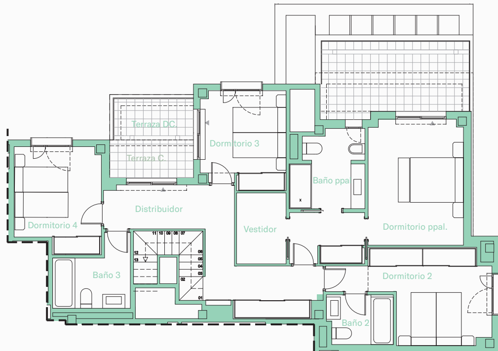
PLANTA SUPERIOR
