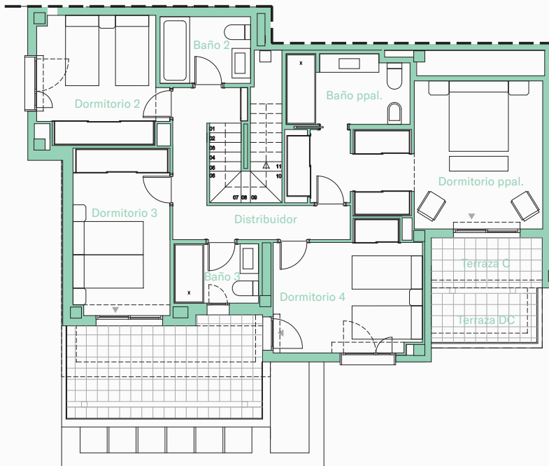
PLANTA INFERIOR
