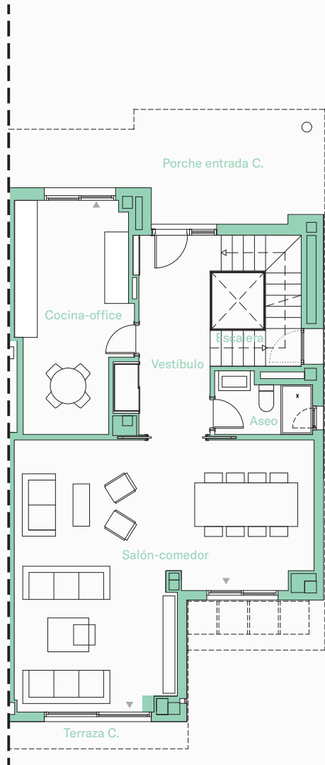
PLANTA BAJA
