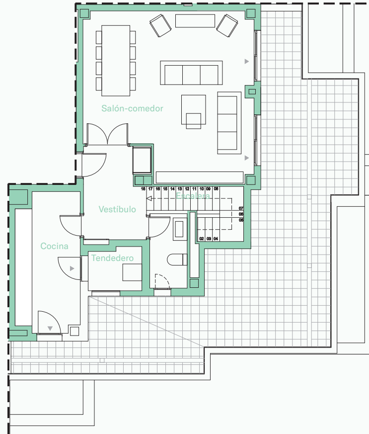
PLANTA SUPERIOR
