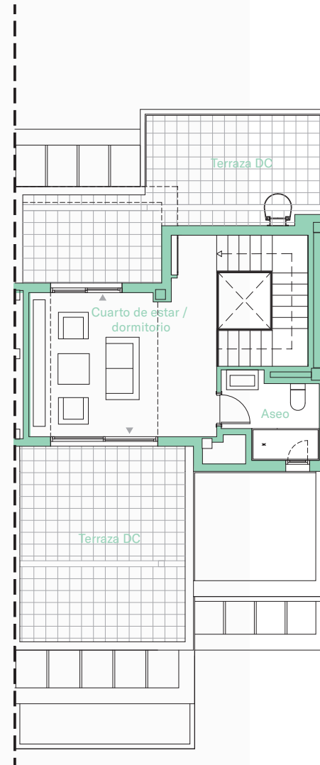
PLANTA SEGUNDA
